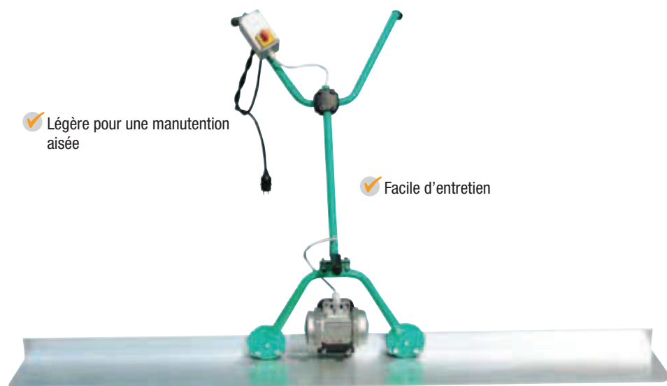
VERSION MONOPHASÉE
